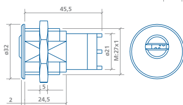
Microconmutador DS-15
