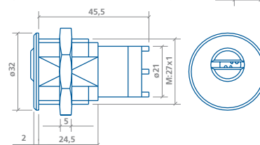
Microconmutador DS-10
