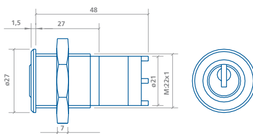
Microconmutador SEA 2 / SEA 3
