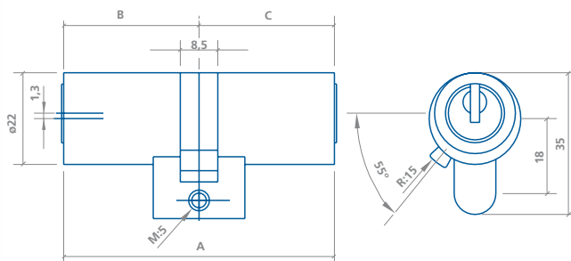
Cilindro SEA 2 / SEA 3
